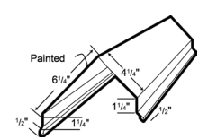
LG 126 DOOR POST TRIM*
