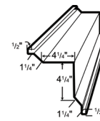
LG 125 9/4" DOOR JAMB
