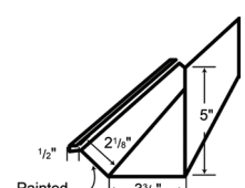
LG 134 TRACK DOOR JAMB TRIM
